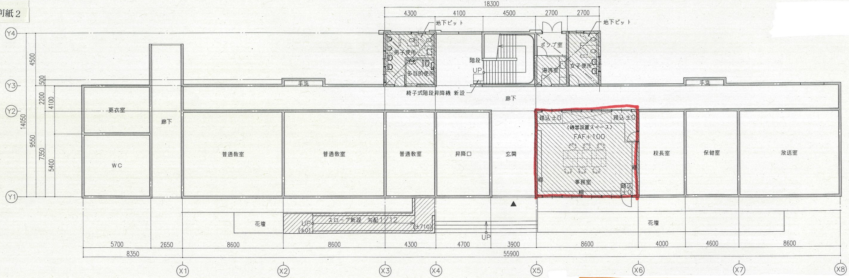
平面図(1階)
