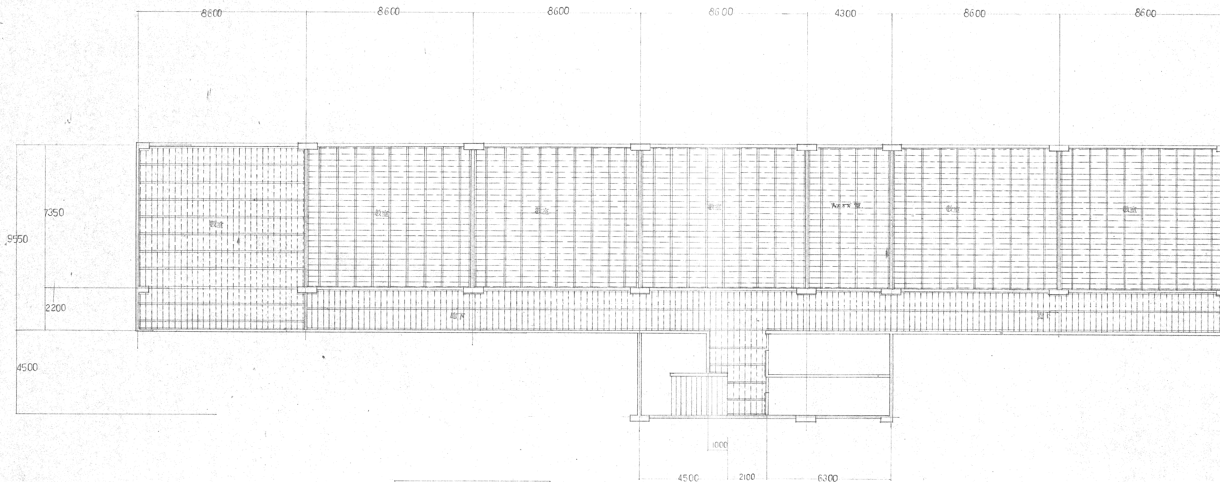
2階床伏図
