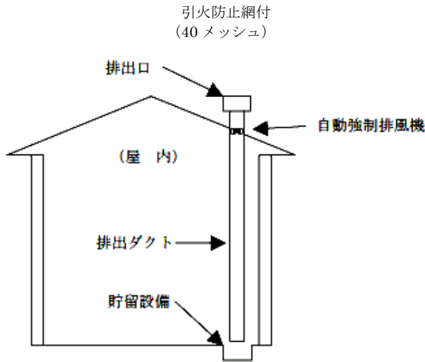
第17-9図 自動強制排出設備の例
