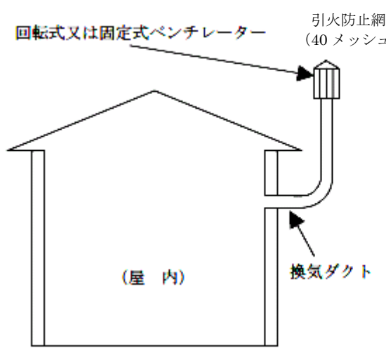
第17- 3 図 強制換気設備の例
