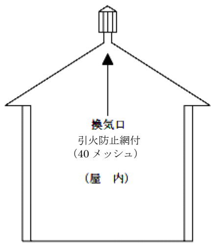
第17- 2 図 強制換気設備の例
