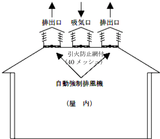
第17-5図 自動強制換気設備の例
