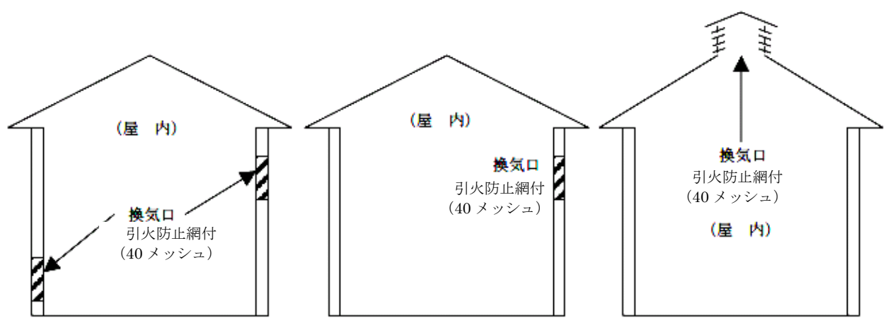
第17- 1 図 自然換気設備の例
