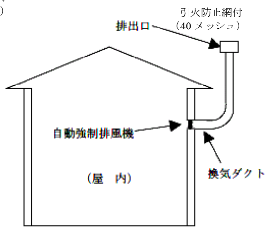
第17- 4 図 自動強制換気設備の例
