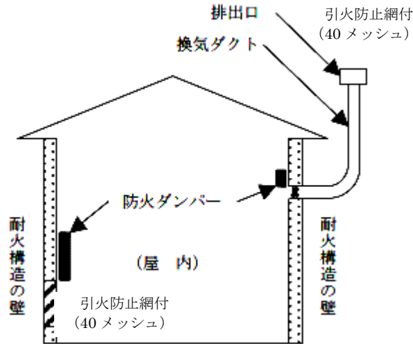
第17-6図 防火ダンパーの設置例
