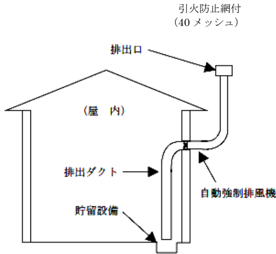
第17-8図 自動強制排出設備の例
