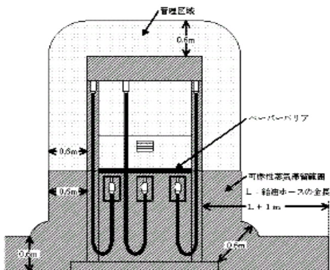
第18－4－2 図 地上式固定給油設備等（可燃性蒸気流入防止構造）
