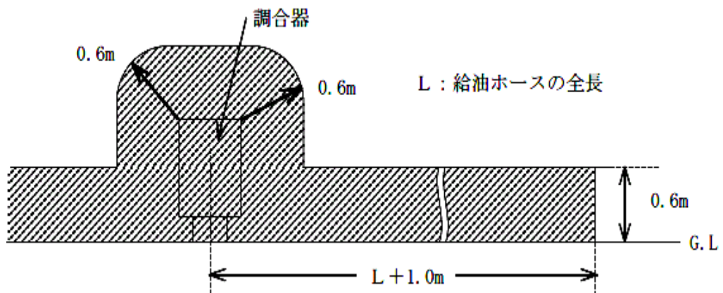
第18-6図 混合燃料調合器
