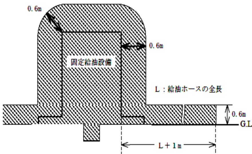
第18－4－1 図 地上式固定給油設備（可燃性蒸気流入防止構造以外）
