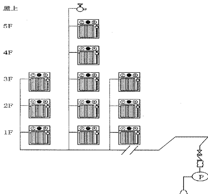
設備概要図
