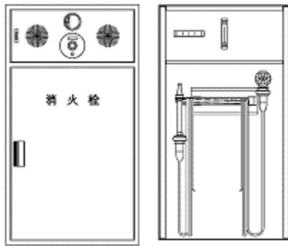
1 号消火栓(易操作性 1 号消火栓を除く。)
