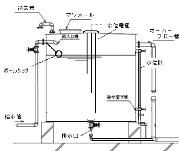
ボールタップを用いるもの
