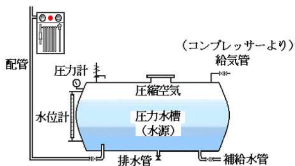
圧力水槽方式の加圧送水装置の構成・系統図
