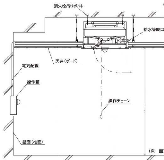
天井設置型消火栓設置例
