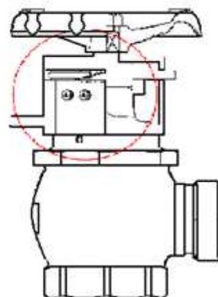
易操作性 1 号消火栓、2 号消火栓又は 広範囲型 2 号消火栓の遠隔起動部
