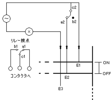
水位電極を用いるもの
