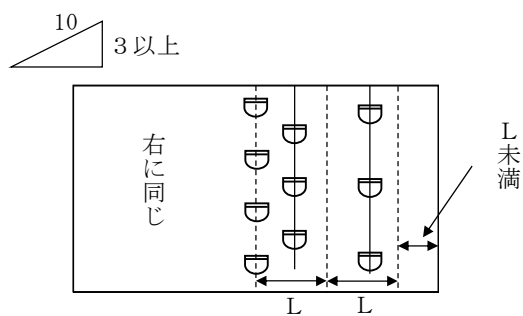
平面図
