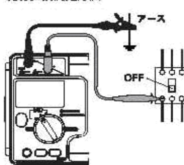
絶縁抵抗測定方法
