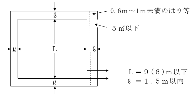
第 11-26 図 差動式分布型（空気管式）
