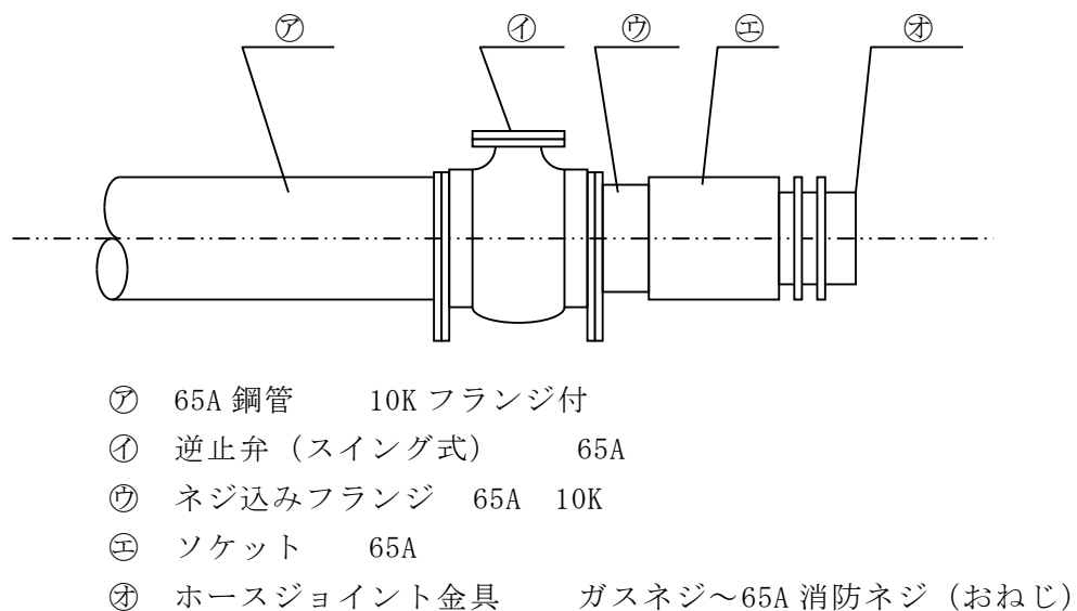
第 6-5 図 放水口
