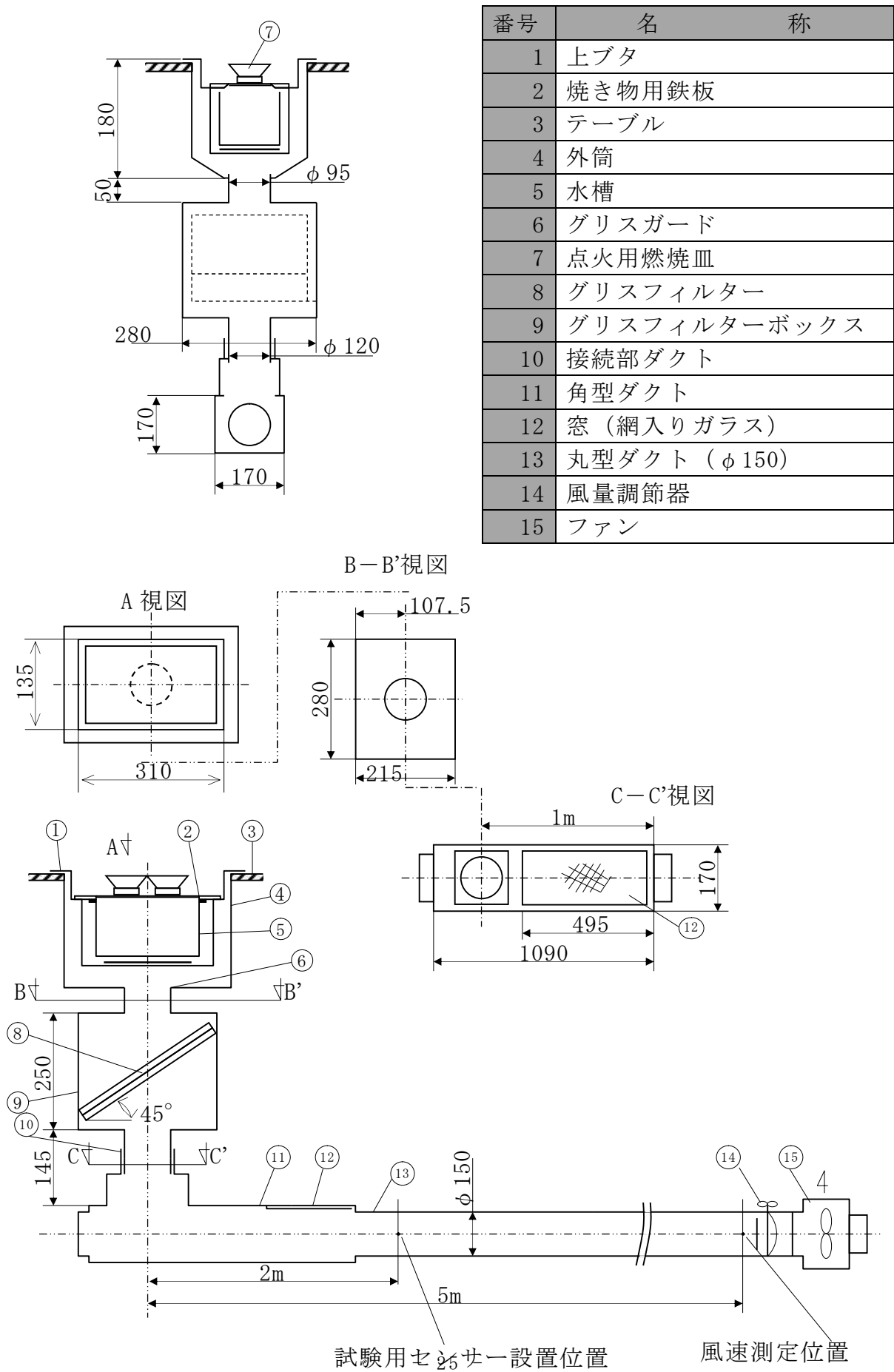
別図2 消火試験図
